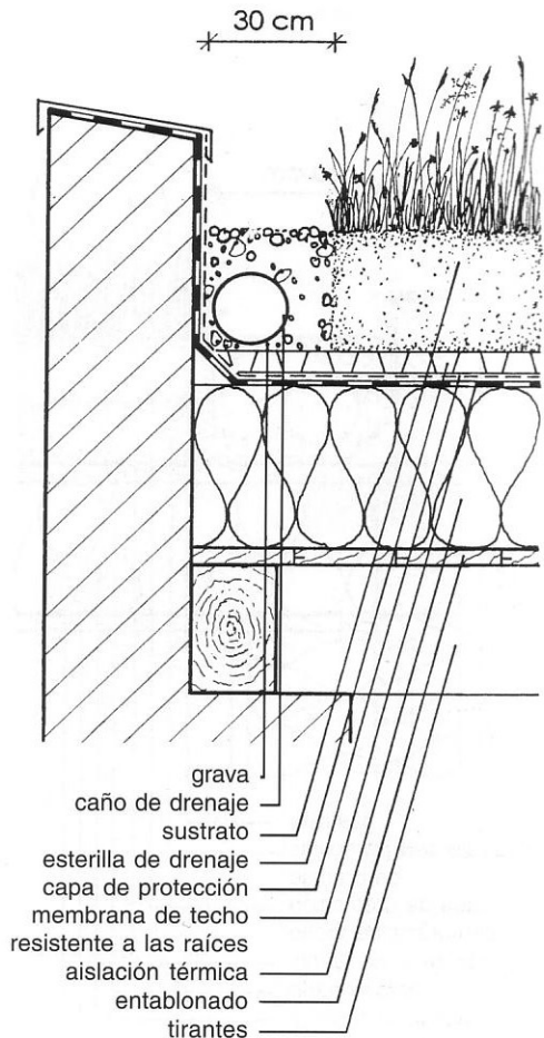
6.5 Conformación de borde de techo con canalón
