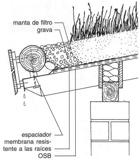
6.11 Detalle de canalón
