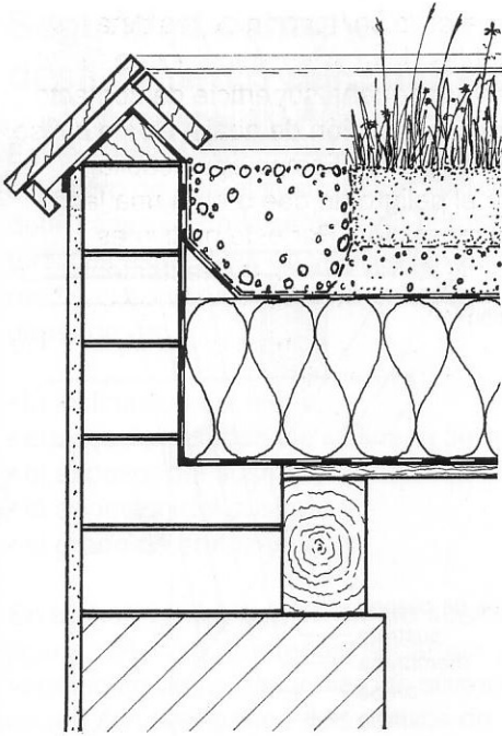
6.8 Detalle de pretil
