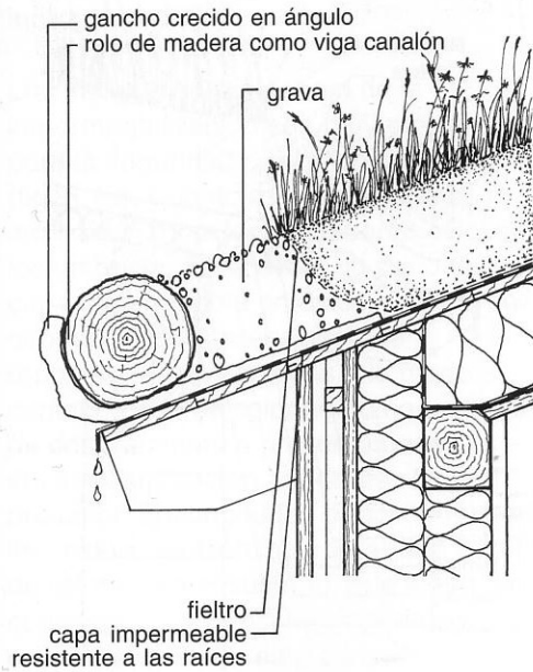
6.10 Detalle de canalón, usado en Escandinavia
