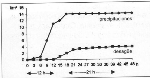
2.11 Volumen de precipitaciones y de desagüe pluvial medidos en un techo verde inclinado después de una lluvia continua de 18 hs de duración (s. Katzschner 1991)
