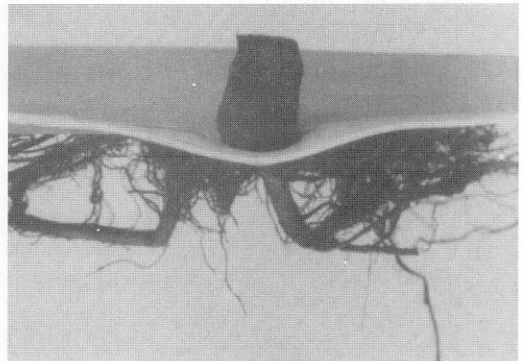
4.6 Perforación en una union pegada de dos láminas de PVC producida por una raíz (Pennigsfeld et al. 1981)
