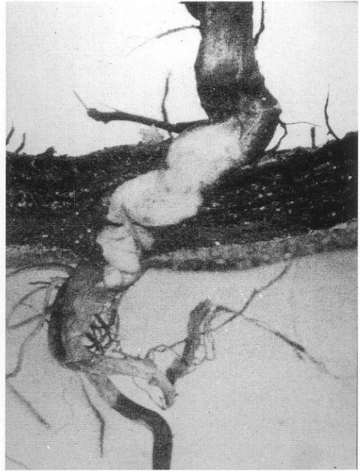
4.5 Perforación producida por raíces de cardos en una membrana asfáltica de cerca de 15mm de espesor, después de 15 meses de duración del ensayo (Pennigsfeld et al. 1981)
